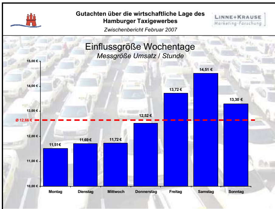
Abb. 17 Einflussgröße Wochentage
